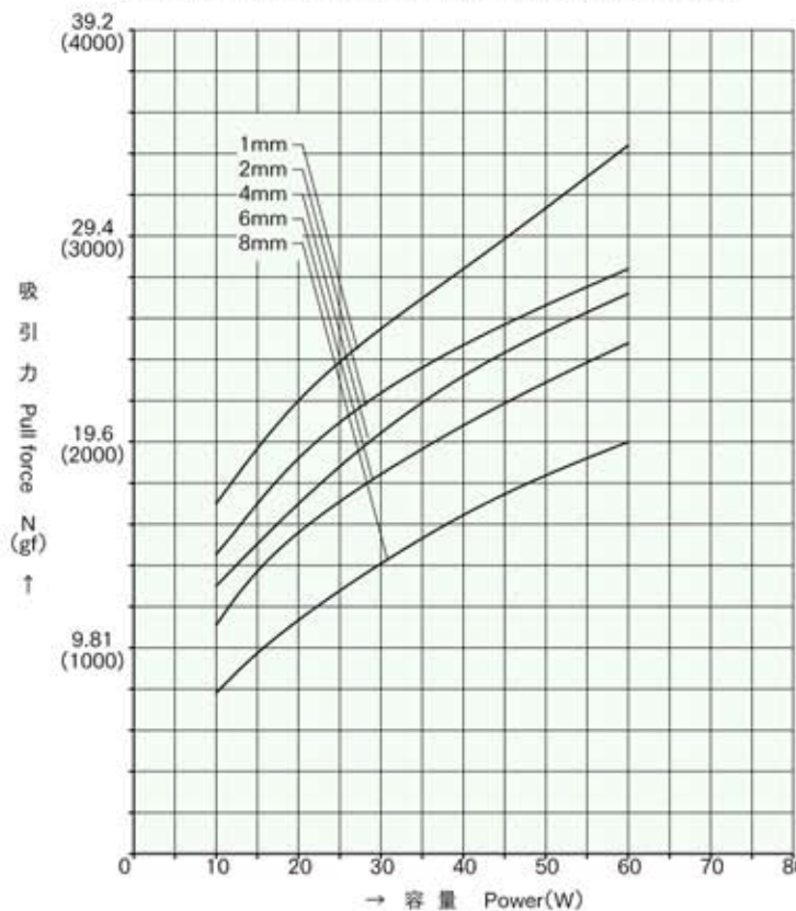
標準コイル表 定格 10W Standard Coil Specifications Rated Power 10W
